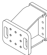
Obrázek 3.11 Distanční držák pro tažné oko stroje, TPL 32
