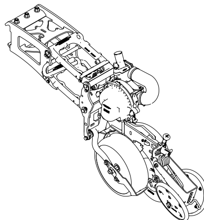
Obrázek 3.17 Výsevní jednotka, dlouhá TPL 32
