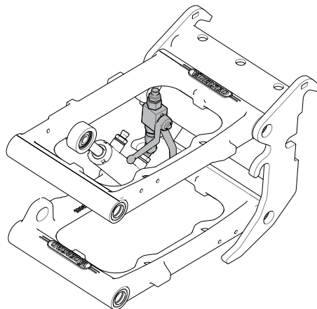
Obrázek 3.10 Kulový ventil pro zajištění výsevní jednotky ve zvednuté poloze, TPL 32
