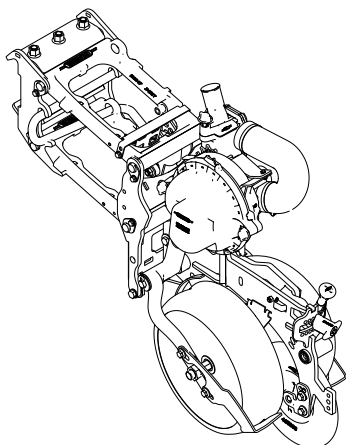
Obrázek 3.18 Výsevní jednotka, krátká TPL 32
