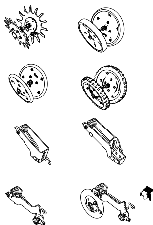
Obrázek 3.19 Zapravovací kola 25, 50, hroty, vzor 50. Rameno zapravovacího kola, pevné krátké nebo nastavitelné dlouhé. TPL 32
