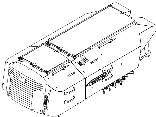
Obrázek 3.14 Zásobník na zrno, Central Fill Combi
