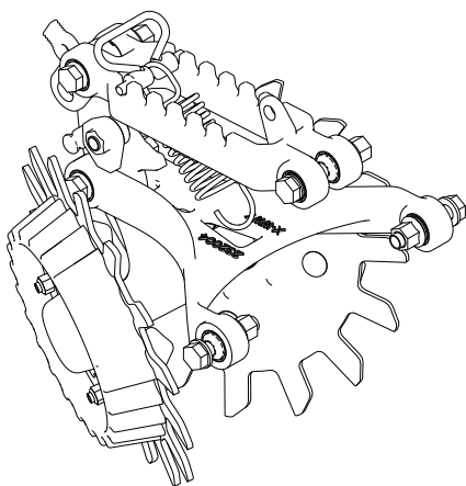
Obrázek 3.20 Čistič řádku, TPL 32
