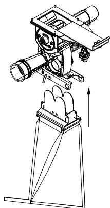
Obrázek 10.30 Nasazení kalibračního sáčku
