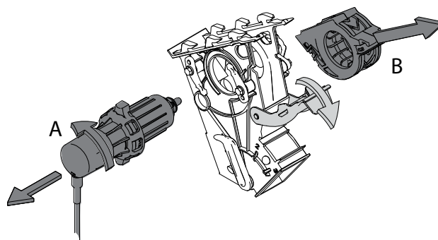
Obrázek 14.32 Demontáž součástí dávkovacího systému pro čištění
