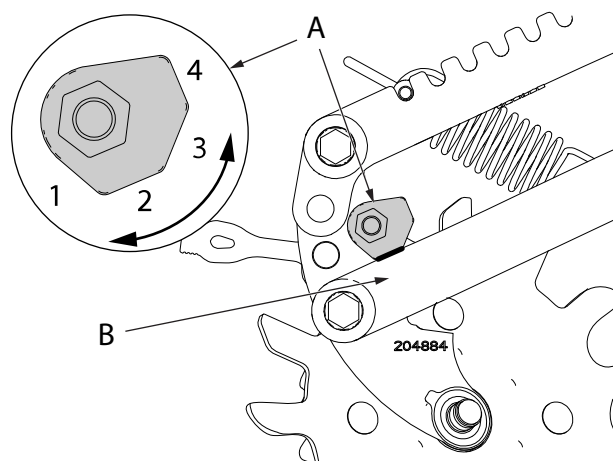
Obrázek 10.28 Polohy spodního dorazu
