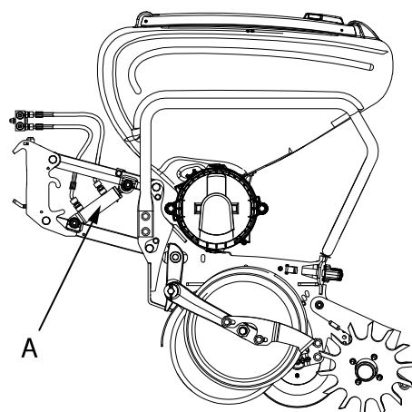
Obrázek 10.19 Hydraulické nastavení přítlaku výsevních jednotek
