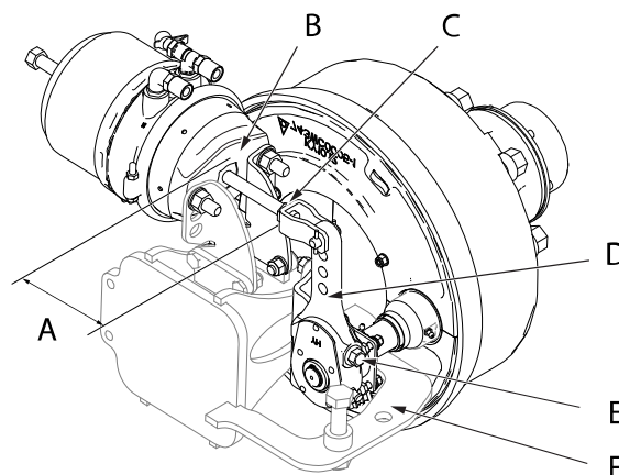
Obrázek 14.37 Délka zdvihu, pneumatické brzdy
