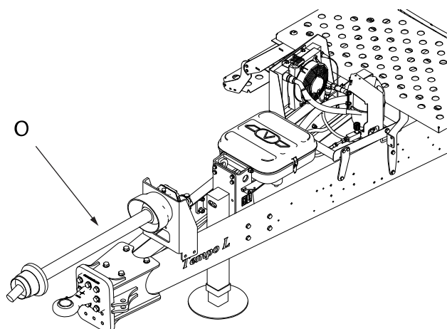
Obrázek 14.59 Vývodový hřídel, PTO
