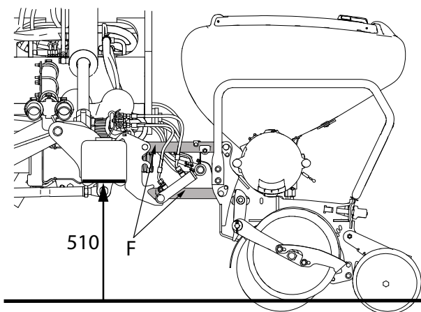
Obrázek 7.3 Paralelogram v horizontální poloze
