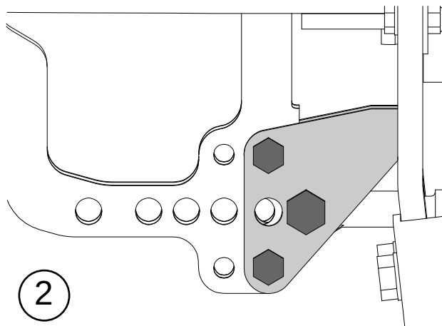
Obrázek 7.13 Zarážka, poloha 2
