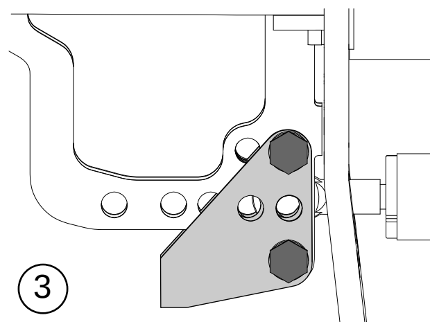
Obrázek 7.14 Zarážka, poloha 3
