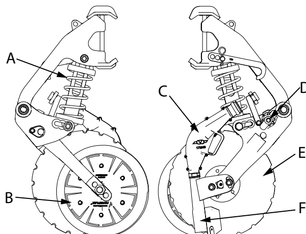
Obrázek 12.9 Přihnojovací jednotka
