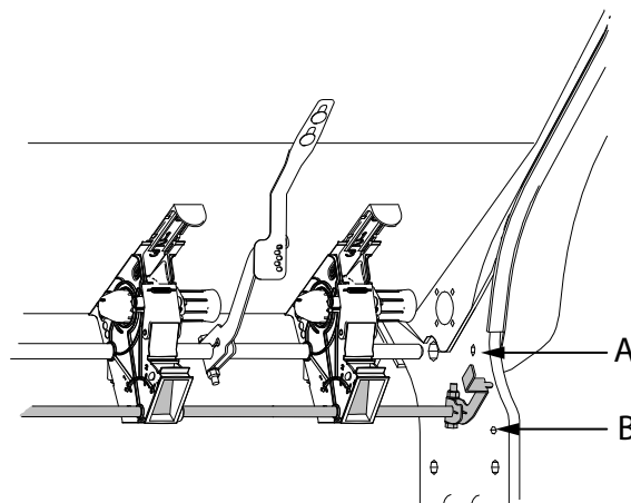
Obrázek 12.6 Kalibrační klapky
