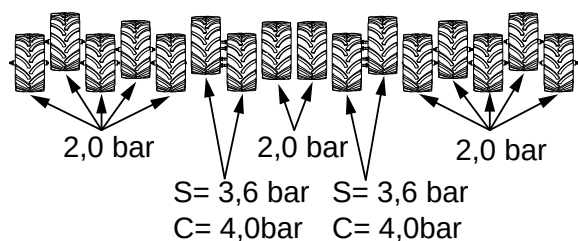
Obrázek 12.36 Kola traktoru
