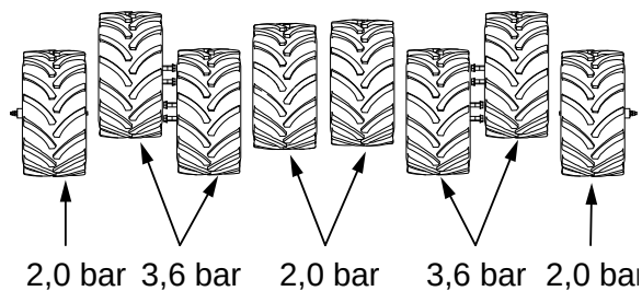
Obrázek 12.34 Kola traktoru
