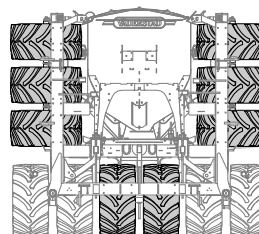
Obrázek 12.32 Hloubkové kolo pěchu
