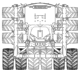
Obrázek 12.33 Hloubkové kolo
