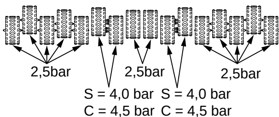
Obrázek 12.40 Kola pro lehké půdy
