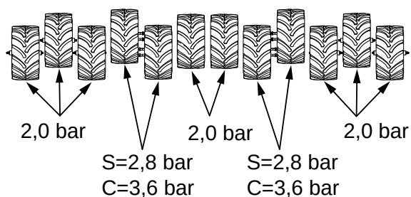
Obrázek 12.35 Kola traktoru
