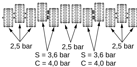
Obrázek 12.39 Kola pro lehké půdy
