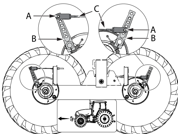
Obrázek 9.21 Carrier XL 925
