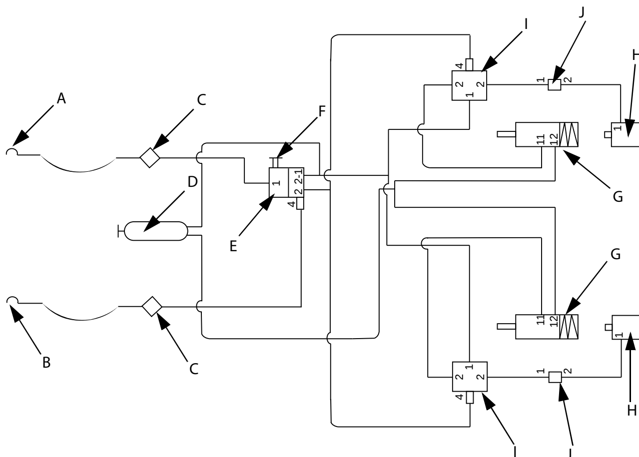
Obrázek 11.2 CRXL 1225
