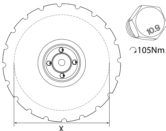
Obrázek 9.12 Jiné kotouče
