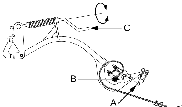
Obrázek 7.7 Kypřicí radlička
