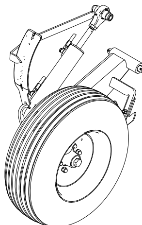
Obrázek 9.21 Standardní opěrné kolo pro SW 560
