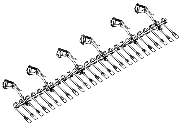
Obrázek 3.4 Kypřič
